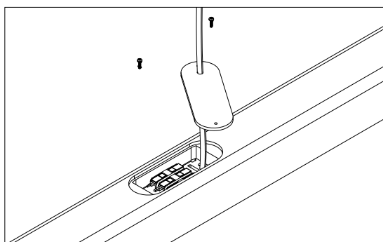
Passer le câble dans la plaque
