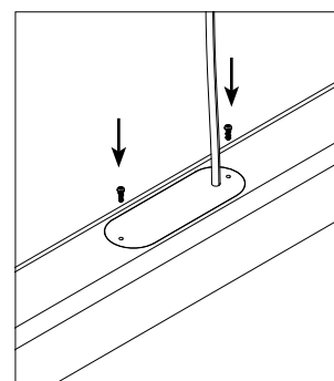
Remettre la plaque Les écritures visibles à l'extérieur
